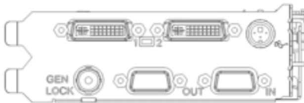
Panneau entrée/sortie de la carte Wildcat III 6210
